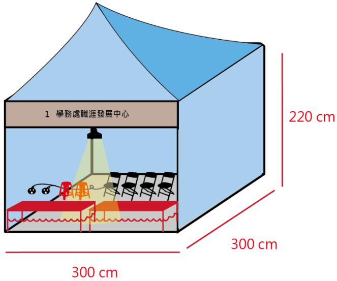
標準單展位圍布平視圖
